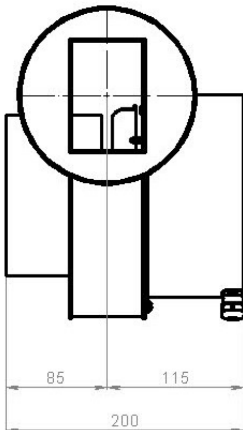
Фигура 2.2. Информация за габаритните и присъединителните размери на вентилаторната група – поглед отгоре ;
