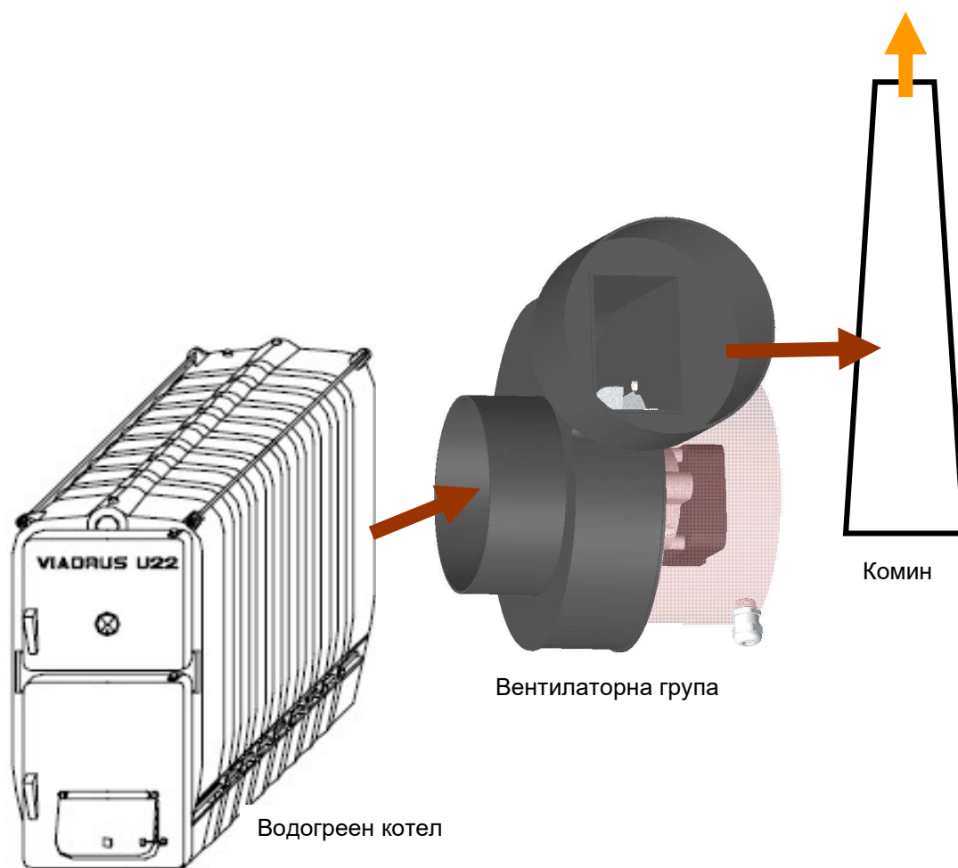
Фигура 4.1. Принципна хидравлична схема за свързване вентилаторната група за принудително отвеждане на димни газове от съоръжение към комин;
