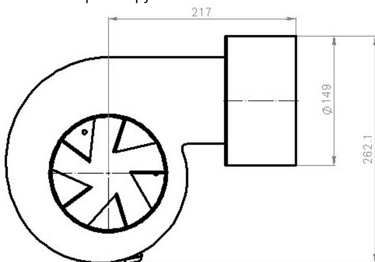
Фигура 2.1. Информация за габаритните и присъединителните размери на вентилаторната група – поглед откъм входящото сечение на модула;
