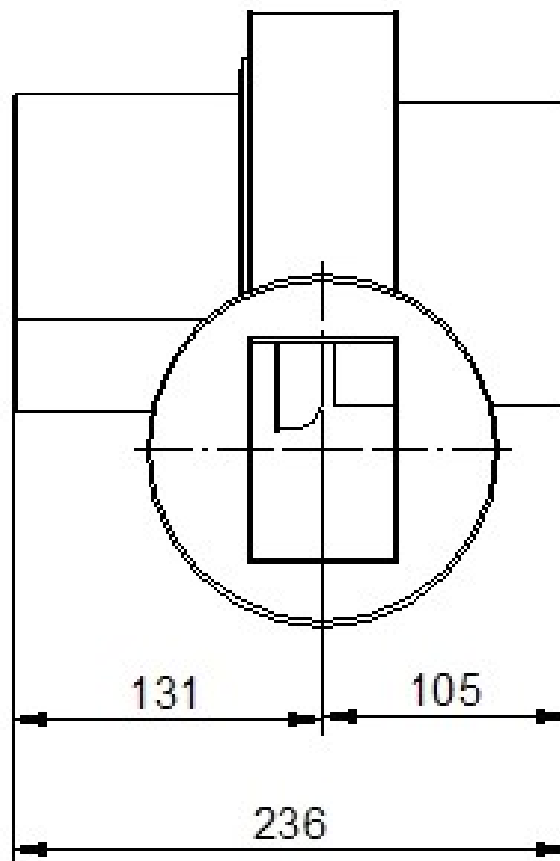
Фигура 2.3. Информация за габаритните и присъединителните размери на вентилаторната група – поглед откъм изходящото сечение на модула ;
