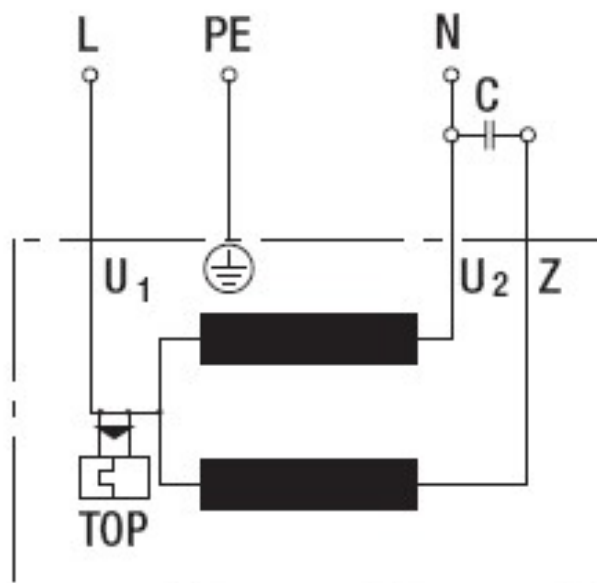
Фигура 6.1. Принципна електрическа схема за свързване на центробежния димосмукателен вентилатор от модула към електрическото захранване;
