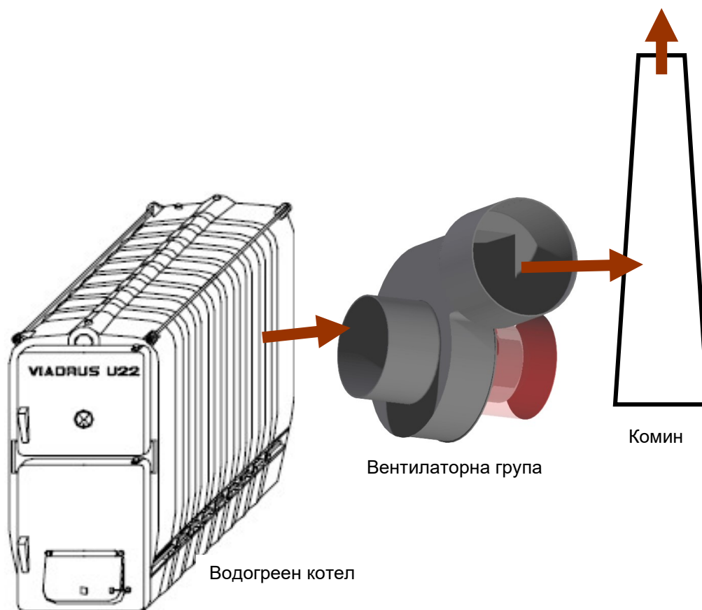
Фигура 4.1. Принципна хидравлична схема за свързване вентилаторната група за принудително отвеждане на димни газове от съоръжение към комин;
