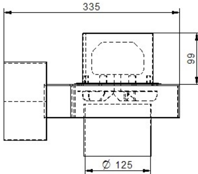
Фигура 2.2. Информация за габаритните и присъединителните размери на вентилаторната група – поглед отгоре ;
