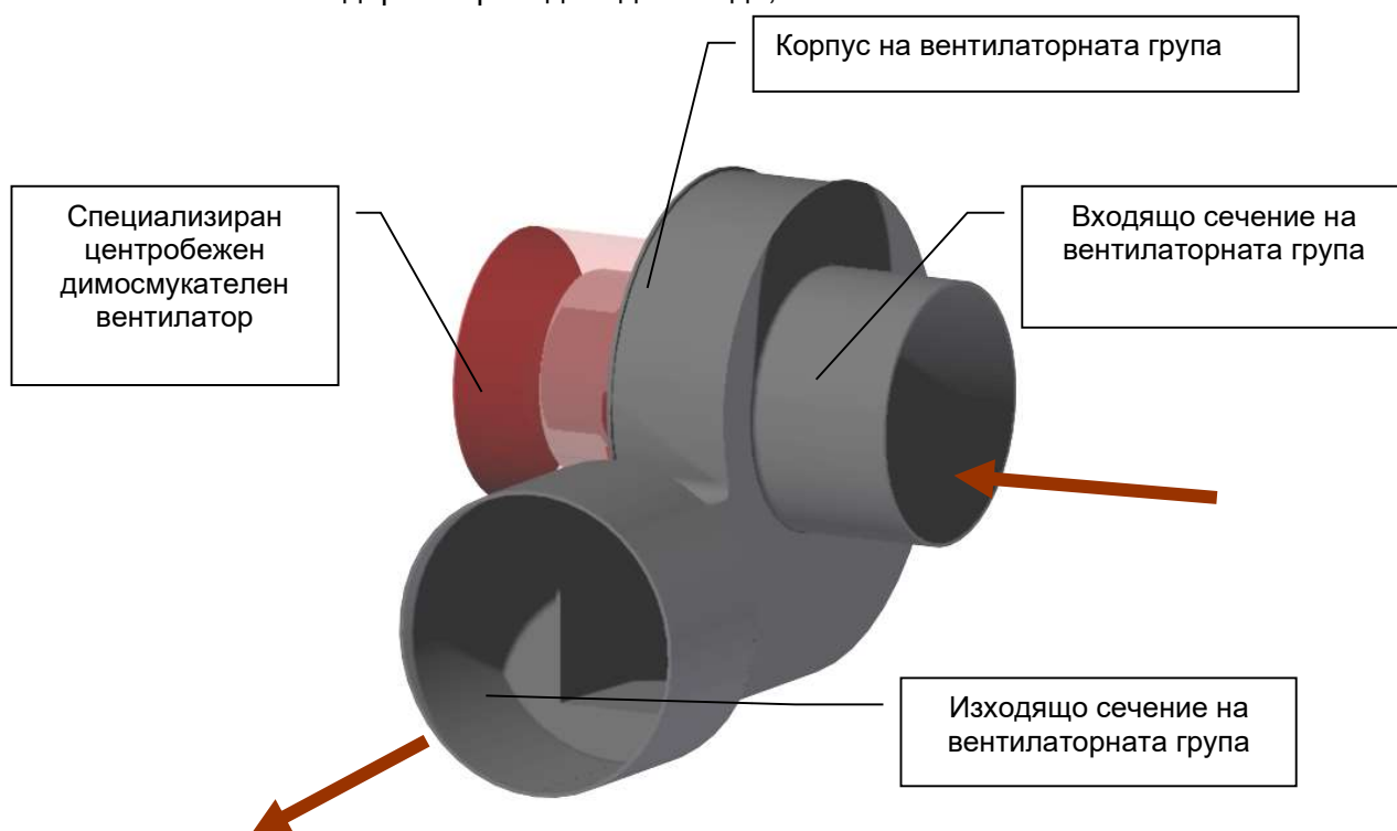
Фигура 3.1. Основни елементи на вентилаторната група за принудително отвеждане на димни газове.
