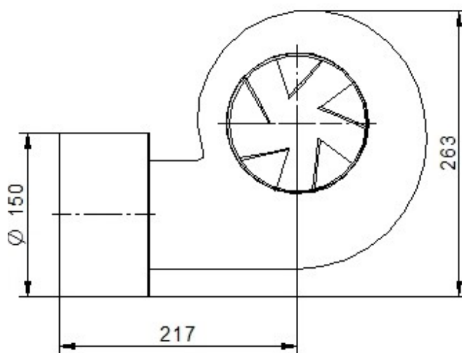
Фигура 2.1. Информация за габаритните и присъединителните размери на вентилаторната група – поглед откъм входящото сечение на модула;
